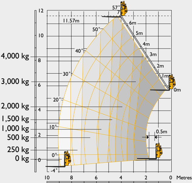
540-170 Estabilizadores retraídos
